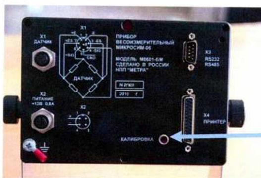
Рисунок 3 - Места пломбирования терминала M0601 для нанесения знака поверки
